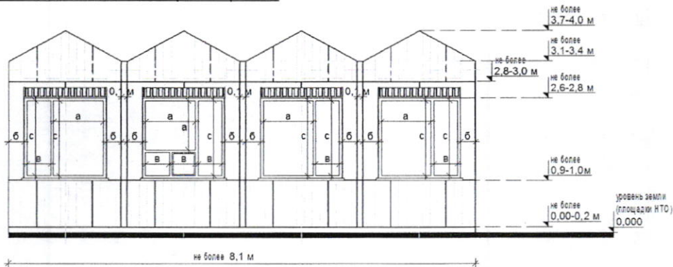
схема с максимальными размерами:
