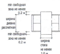
четырёхместное размещение:
