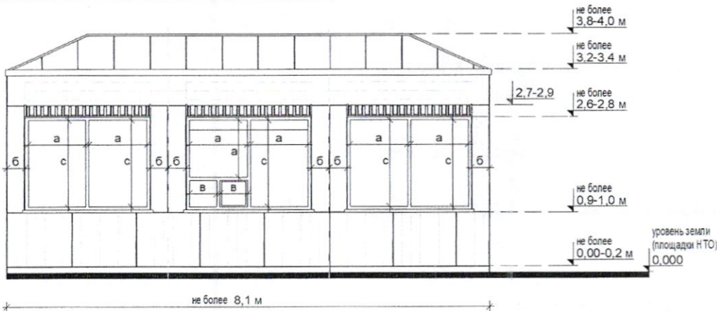
ВИД 3
