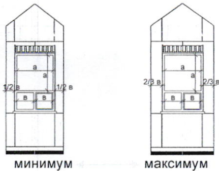
схема допустимого увеличения простенков:
