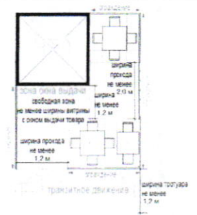
площадка сезонного (летнего) кафе до 10 мест с киоском без технологического настила, двухрядное размещение:
