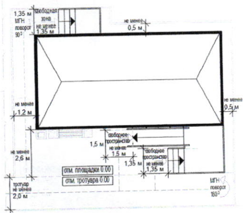
схемы места размещения нестационарного торгового объекта при размещении павильона на Т-образном перекрестке тротуаров:
