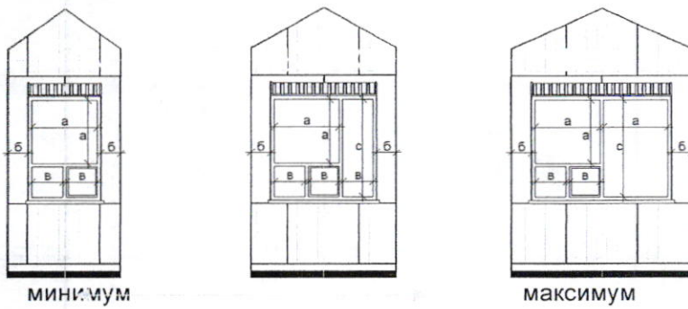
схема допустимого увеличения простенков:
