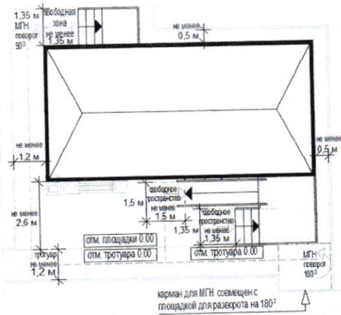
схемы места размещения нестационарного торгового объекта при размещении павильона на Т-образном перекрестке тротуаров:
