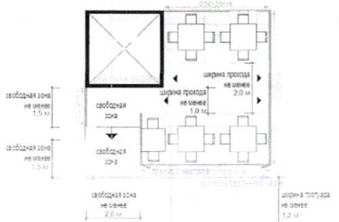
площадка сезонного (летнего) кафе 10-26 мест с павильоном и технологическим настилом, двухрядное размещение:
