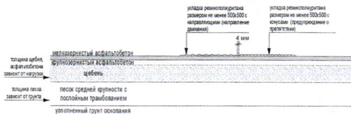
схема сопряжения существующего тротуара, тактильного покрытия:
