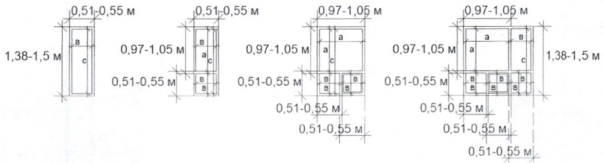
схема допустимого увеличения площади остекления:
