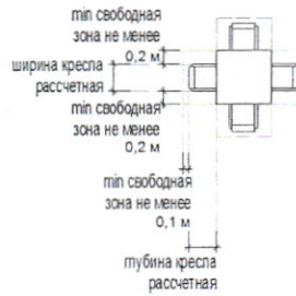
четырёхместное размещение:
