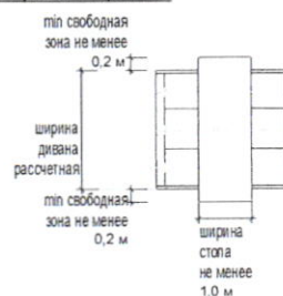
шестиместное размещение:
